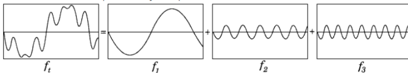
GAMBAR 1. Ilustrasi penjumlahan beberapa sinyal sinusoidal
