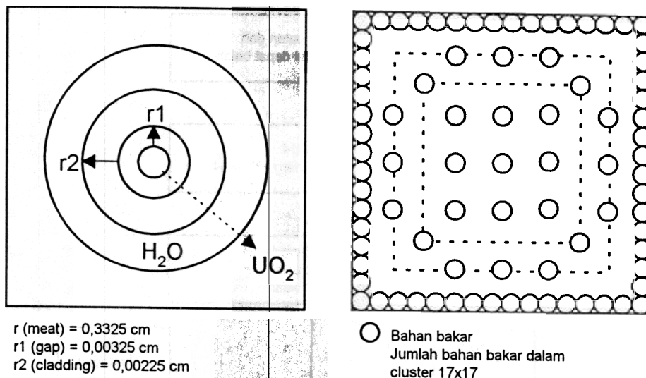
Gambar 3. Pemodelan sel teras AP-600
