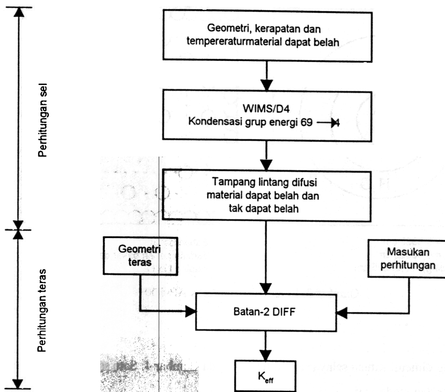
Gambar 2. Diagram alir perhitungan
