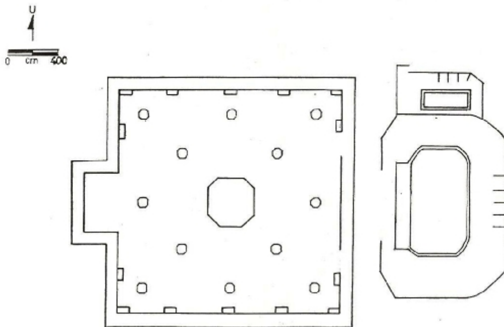
Gambar 4. Denah Masjid Raya Tanjung Pauh Hilir
