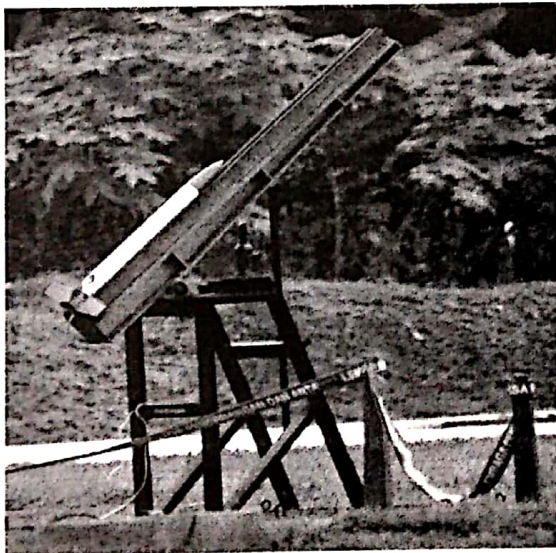
Gambar 2-2: Roket LOCON dgn peluncurnya
