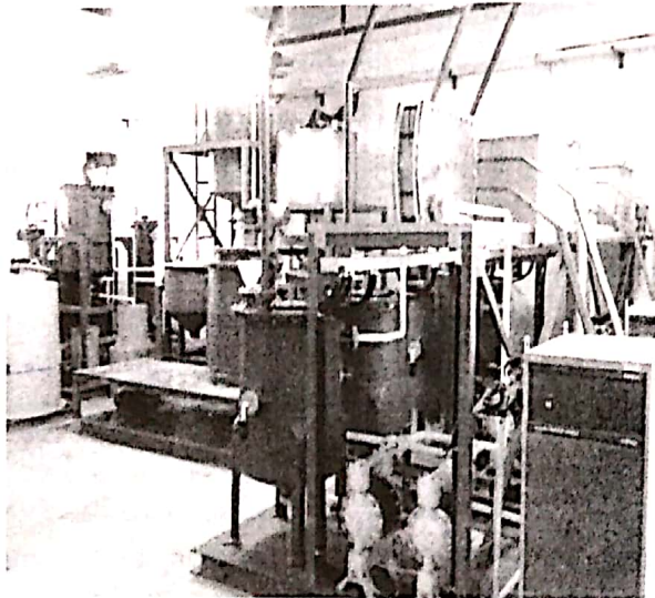
Gambar 3-1: Sel Elektrolisis \text{NaCl} menjadi \text{NaClO}_4
