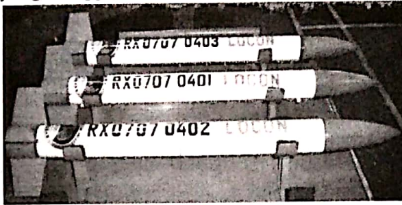
Gambar 2-1: Roket LOCON siap terbang
