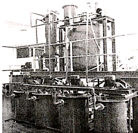
Gambar 4-1: Rangkaian alat pemurnian NaCl
