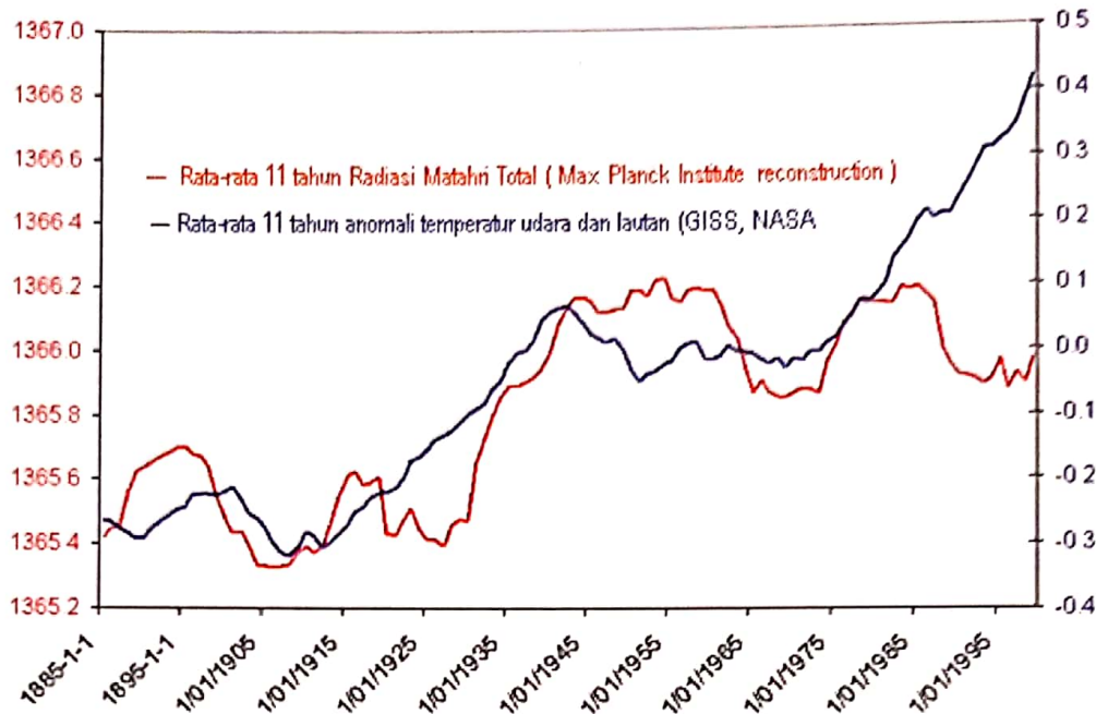
Gambar 3-1: Radiasi Matahari Total dan Temperatur Global 1885 – 2000 (Sumber Max Planck dan NASA)
