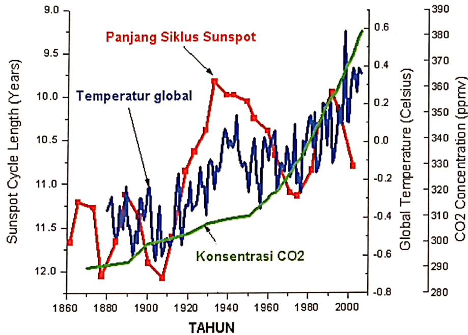
Gambar 2-1: Kenaikan Temperatur Global, Konsentrasi CO 2 dan Siklus Sunspot (dikompilasi oleh Gregory, 2010)
