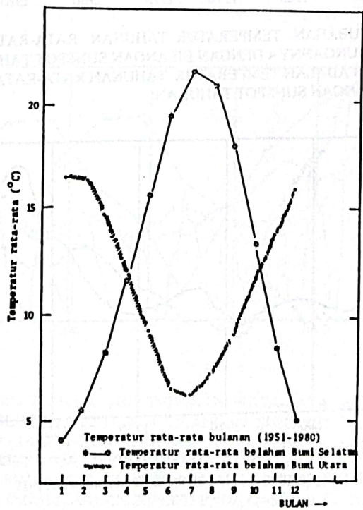
Gambar 3.2 : PERUBAHAN TEMPERATUR RATA-RATA BULANAN UNTUK BELAHAN BUMI UTARA DAN BELAHAN BUMI SELATAN.
