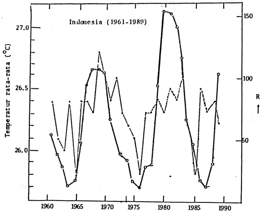
Gambar 3.3: PERUBAHAN TEMPERATUR TAHUNAN RATA-RATA INDONESIA DAN HUBUNGANNYA DENGAN BILANGAN SUNSPOT TAHUNAN. GARIS-GARIS TIPIS ADALAH TEMPERATUR TAHUNAN RATA-RATA DAN GARIS TEBAL BILANGAN SUNSPOT TAHUNAN.
