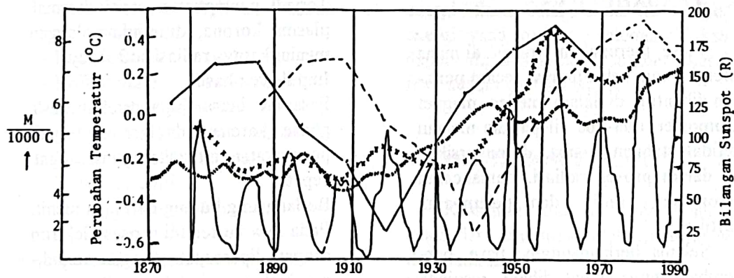
Gambar 3.6 : SIMPANGAN TEMPERATUR TAHUNAN RATA-RATA, BILANGAN SUNSPOT, MOVING SEGMENT 22 TAHUN BILANGAN SUNSPOT DAN PERIODE KURVA ROTASI 100 TAHUN. KURVA ROTASI DIGAMBARKAN DENGAN GARIS PENUH DAN PUTUS-PUTUS, SEDANGKAN MOVING SEGMENT 22 TAHUN BILANGAN SUNSPOT, SIMPANGAN TEMPERATUR RATA-RATA, DAN BILANGAN SUNSPOT TAHUNAN DIGAMBARKAN SEPERTI PADA GAMBAR 3.4 DAN 3.5.
