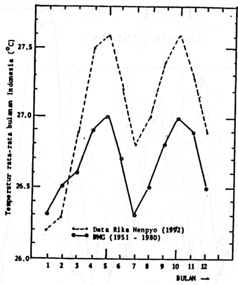
Gambar 3.1 : PERUBAHAN TEMPERATUR RATA-RATA BULANAN
