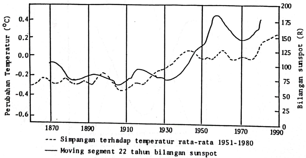
Gambar 3.4: SIMPANGAN TEMPERATUR RATA-RATA TAHUNAN DINORMALISASI TERHADAP TEMPERATUR RATA-RATA DARI TAHUN 1951 SAMPAI DENGAN 1980 DAN MOVING SEGMENT 22 TAHUN BILANGAN SUNSPOT.
