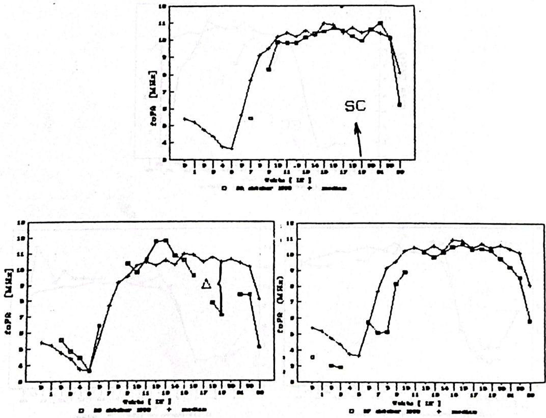
Gambar 3.10 : foF2 TANGGAL 25, 26, DAN 27 OKTOBER 1993 DAN MEDIAN BULANAN DI ATAS SPD-BIAK.
