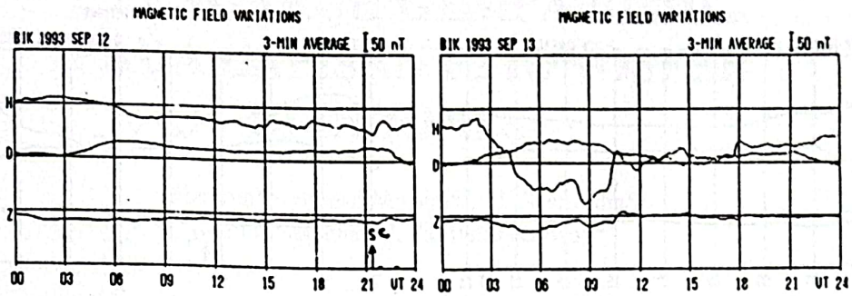
Gambar 3.7 : VARIASI MEDAN MAGNET BUMI TANGGAL 12 DAN 13 SEPTEMBER 1993 DI SPD BIAK.
