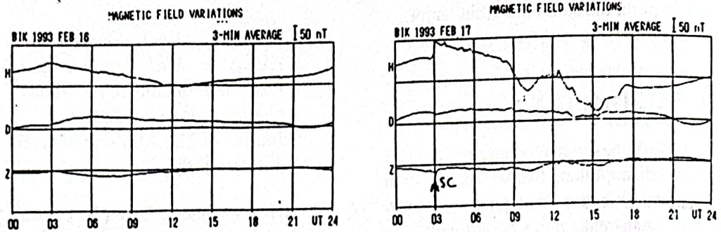
Gambar 3.1 : VARIASI MEDAN MAGNET BUMI TANGGAL 16 DAN 17 FEBRUARI 1993 DI SPD BIAK.
