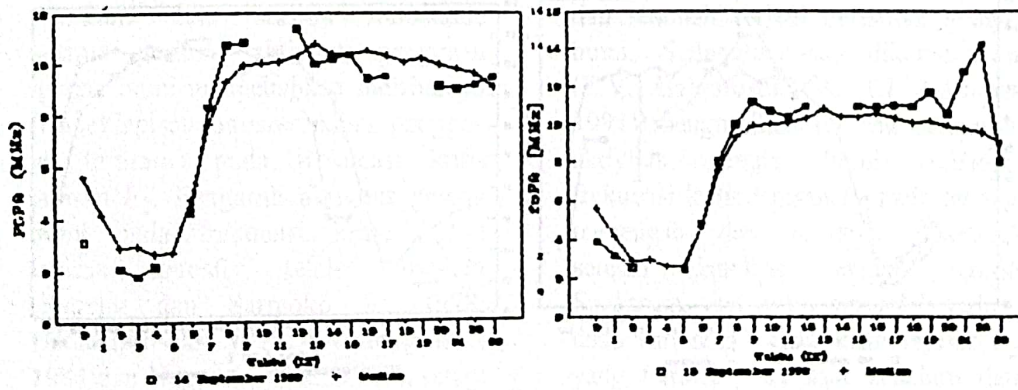
Gambar 3.8 : foF2 TANGGAL 13, 14, DAN 15 SEPTEMBER 1993 DAN MEDIAN BULANAN DI ATAS SPD BIAK.
