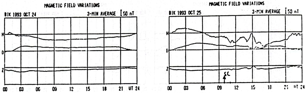
Gambar 3.9 : VARIASI MEDAN MAGNET BUMI TANGGAL 24 DAN 25 OKTOBER 1993 DI SPD BIAK.
