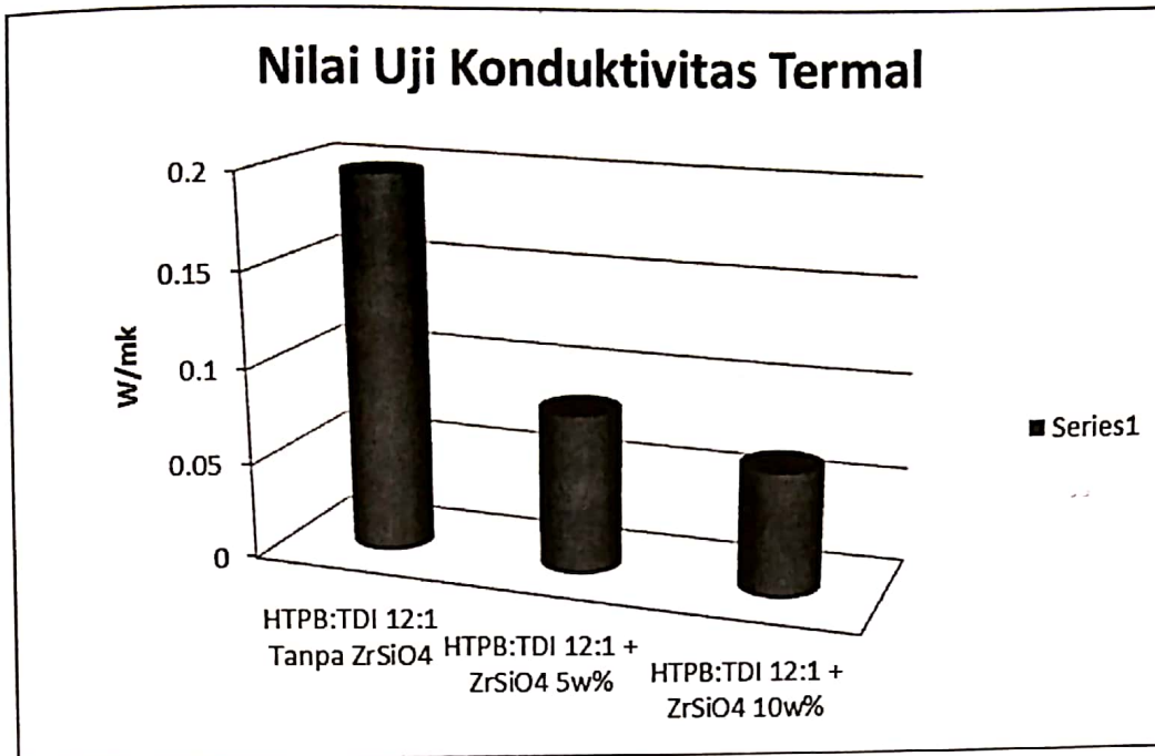
Gambar 4-1: Grafik Nilai Konduktivitas Termal Liner
