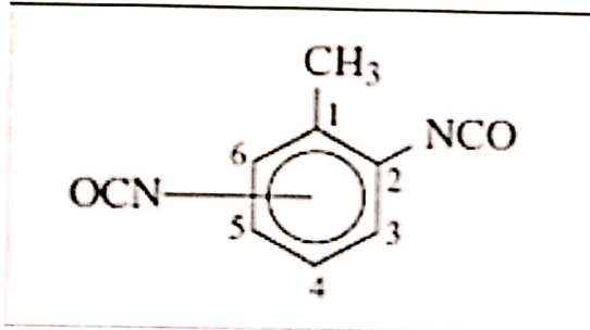
Gambar 2-2: Struktur Molekul TDI
