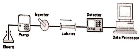
Gambar 5-1: Rangkaian dasar komponen kromatografi
