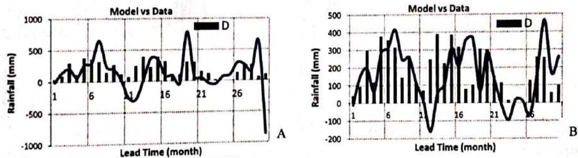
Gambar 3-5: Perbandingan hasil prakiraan (model) dan pengamatan (data) dengan nilai dimensi embedding 25 dan korelasi 0,36 (A) dan nilai dimensi embedding 26 dan korelasi 0,42 (B)
