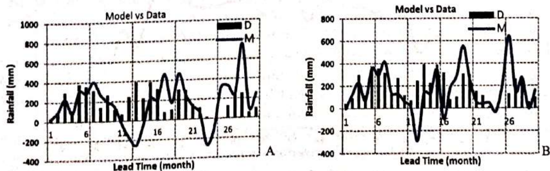
Gambar 3-6: Perbandingan hasil prakiraan (model) dan pengamatan (data) dengan nilai dimensi embedding 27 dan korelasi 0,25 (A) dan nilai dimensi embedding 28 dan korelasi 0,34 (B)
