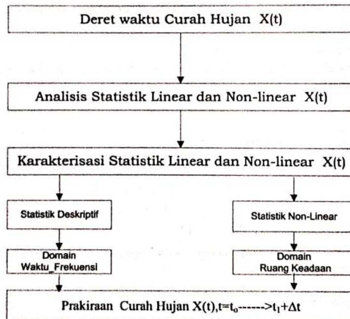
Gambar 2-4: Diagram alir pengolahan dan prakiraan data curah hujan di area Situ Cileunca
