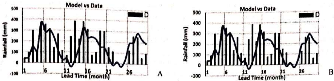
Gambar 3-3: Perbandingan hasil prakiraan (model) dan pengamatan (data) dengan nilai dimensi embedding 21 dan korelasi 0,52 (A) dan nilai dimensi embedding 22 dan korelasi 0,56 (B)
