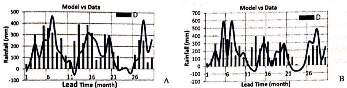
Gambar 3-4: Perbandingan hasil prakiraan (model) dan pengamatan (data) dengan nilai dimensi embedding 23 dan korelasi 0,60 (A) dan nilai dimensi embedding 24 dan korelasi 0,52 (B)
