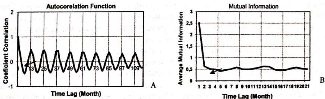
Gambar 3-2: Fungsi Autokorelasi (A) dan Informasi mutual (B) untuk data curah hujan bulanan untuk mencari waktu tunda ( lag time ) saat jatuh mendekati 0
