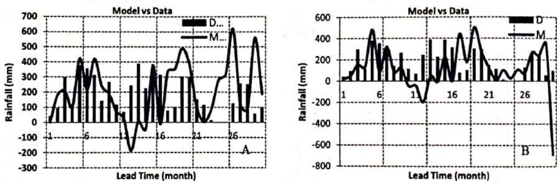
Gambar 3-7: Perbandingan hasil prakiraan (model) dan pengamatan (data) dengan nilai dimensi embedding 29 dan korelasi 0,025 (A) dan nilai dimensi embedding 30 dan korelasi 0,29 (B)
