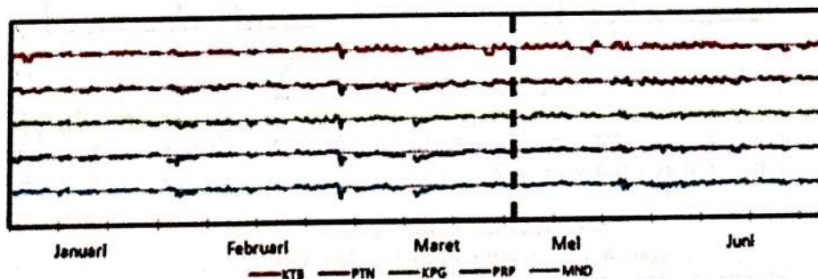
Gambar 3-4c:Gangguan geomagnet dari ke 5 stasiun (Kototabang-KTB, Pontianak-PTN, Kupang-KPG, Parepare-PRP, dan Manado-MND) regional Indonesia pada rentang waktu tahun 2011 setelah distandarisasi
