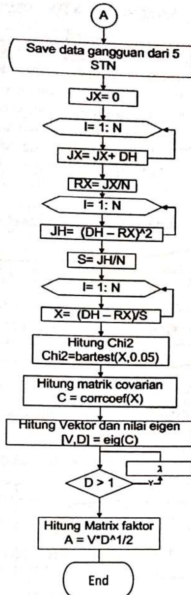
Gambar 2-2: Diagram alir dari pengolahan data gangguan geomagnet regional Indonesia dengan metode analisis komponen utama ( Principal Component Analysis/PCA )
