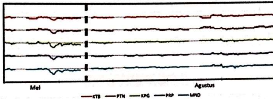
Gambar 3-4b:Gangguan geomagnet dari ke 5 stasiun (Kototabang-KTB, Pontianak-PTN, Kupang-KPG, Parepare-PRP, dan Manado-MND) regional Indonesia pada rentang waktu tahun 2010 setelah distandarisasi
