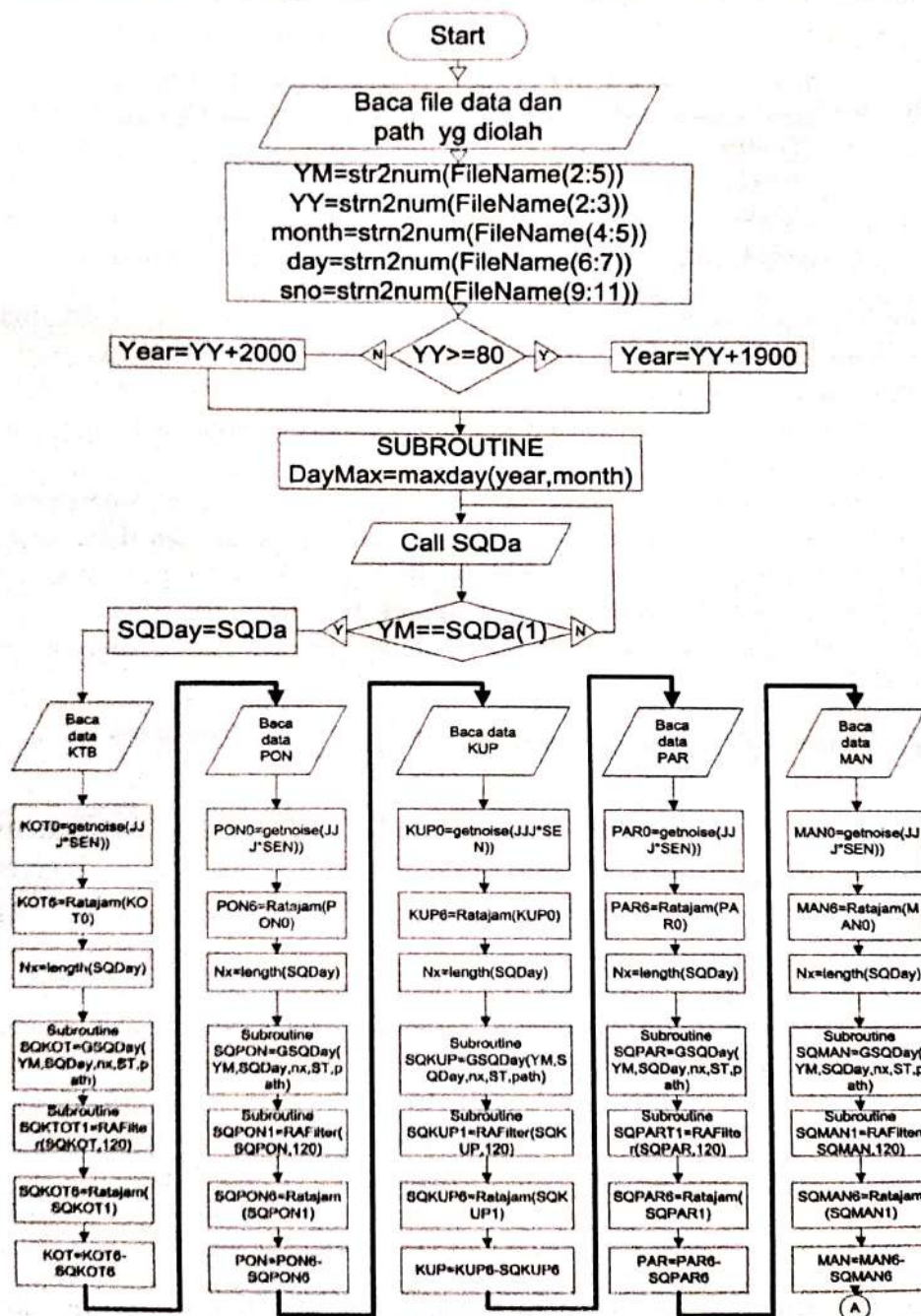
Gambar 2-1: Diagram alir pengolahan gangguan geomagnet dari 5 stasiun
