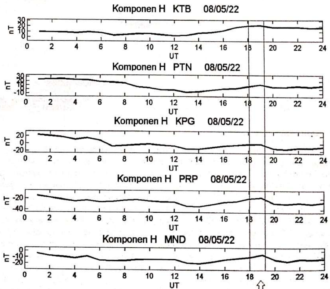
Gambar 3-2: Variasi gangguan geomagnet dari 5 stasiun (Kototabang-KTB, Pontianak-PTN, Kupang-KPG, Parepare-PRP, dan Manado-MND) yang berada di regional Indonesia untuk tanggal 22 Mei 2008. Tanda panah menunjukkan waktu terjadinya gangguan geomagnet
