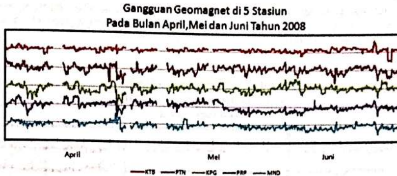
Gambar 3-3a: Gangguan geomagnet dari ke 5 stasiun (Kototabang-KTB, Pontianak-PTN, Kupang-KPG, Parepare-PRP, dan Manado-MND) regional Indonesia tahun 2008 untuk periode waktu seperti pada Tabel 2-2
