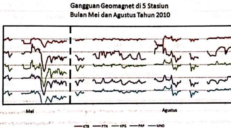
Gambar 3-3b: Gangguan geomagnet dari ke 5 stasiun (Kototabang-KTB, Pontianak-PTN, Kupang-KPG, Parepare-PRP, dan Manado-MND) regional Indonesia tahun 2010 untuk periode waktu seperti pada Tabel 2-2
