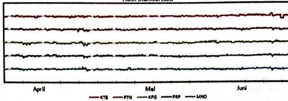
Gambar 3-4a:Gangguan geomagnet dari ke 5 stasiun (Kototabang-KTB, Pontianak-PTN, Kupang-KPG, Parepare-PRP, dan Manado-MND) regional Indonesia pada rentang waktu tahun 2008 setelah distandarisasi
