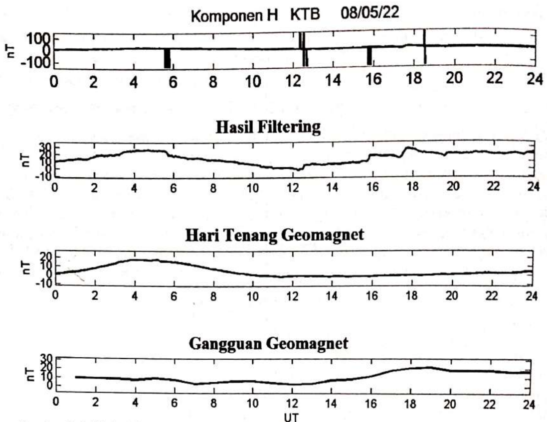
Gambar 3-1: Variasi harian dari Kototabang (KTB) pada tanggal 22 Mei 2008 dan gangguannya
