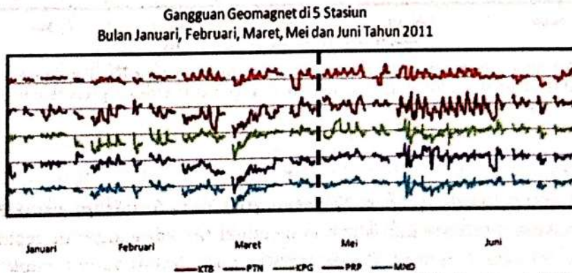
Gambar 3-3c: Gangguan geomagnet dari ke 5 stasiun (Kototabang-KTB, Pontianak-PTN, Kupang-KPG, Parepare-PRP, dan Manado-MND) regional Indonesia tahun 2011 untuk periode waktu seperti pada Tabel 2-2
