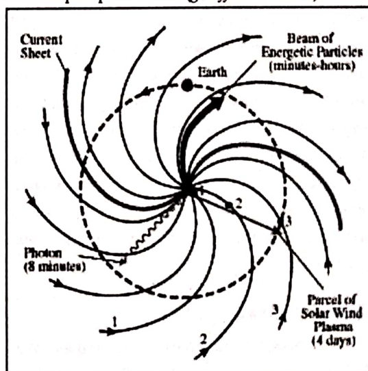
Gambar 3-4: Pola spiral medan magnet dari matahari (Sumber: NASA's Cosmos)
