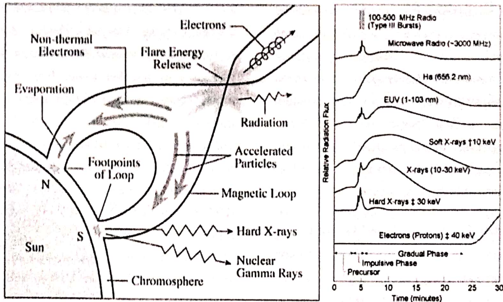
Gambar 3-1: Model pelepasan energi dalam flare (kiri), yang menghasilkan partikel dan radiasi dalam berbagai panjang gelombang (Sumber: NASA's Cosmos)
