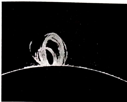
Gambar 3-3: Lengkungan prominens yang menghubungkan medan magnet di korona matahari (Sumber: NASA's Cosmos)
