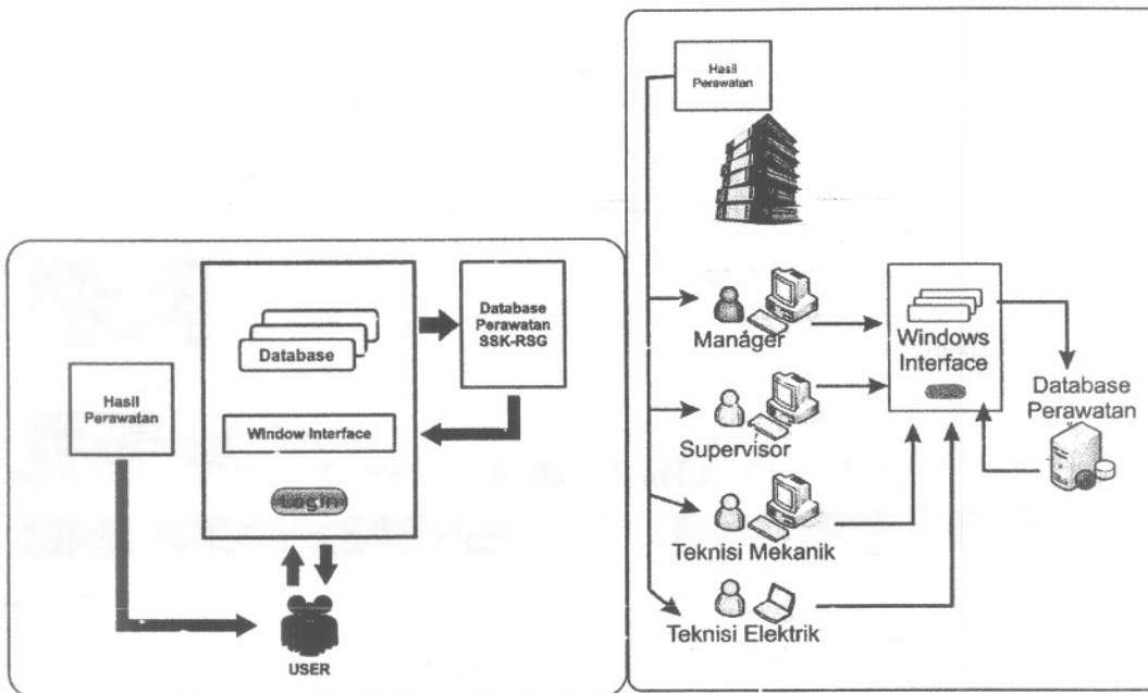
Gambar 6. Ilustrasi hasil pengembangan database perawatan korektif
