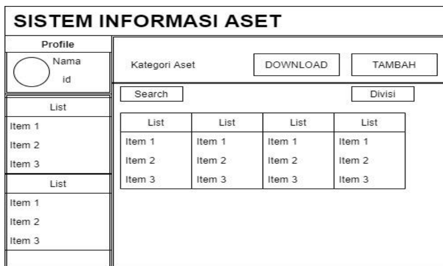
Gambar 11. Halaman kategori aset dan tambah kategori aset antarmuka website .
