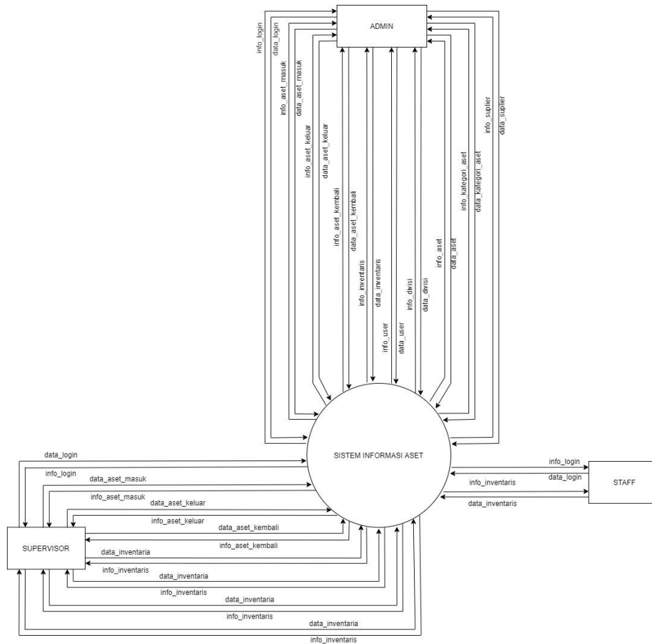
Gambar 2. Diagram konteks
