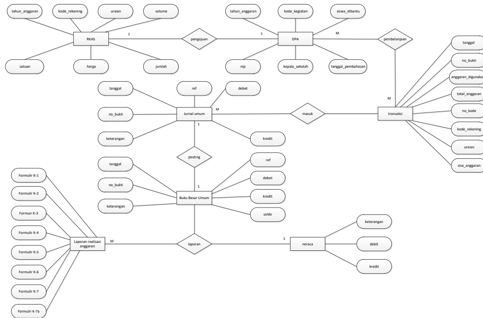
Gambar 5 Entity Relationship Diagram yang Diusulkan
