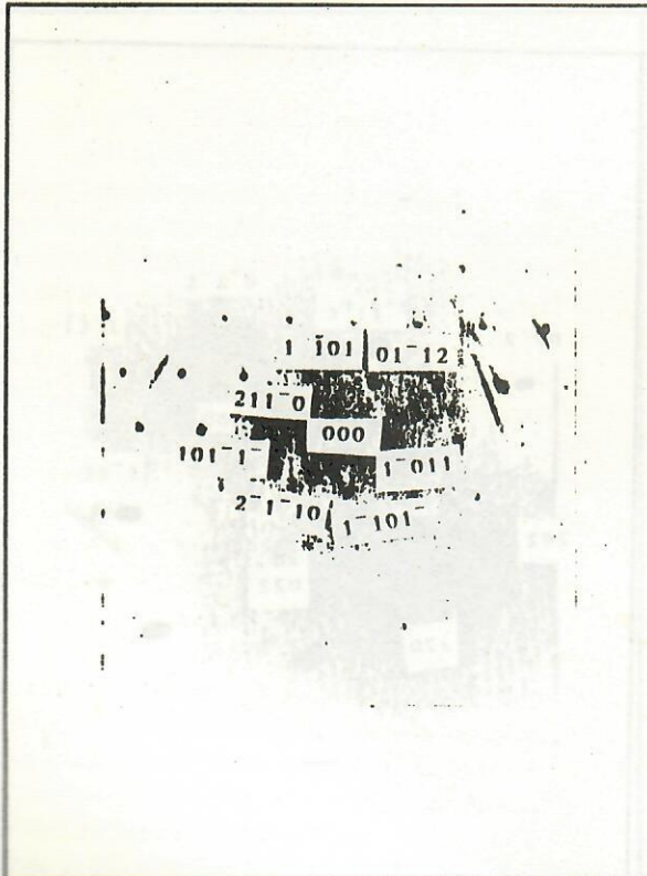
Gambar 6.a. Pola difraksi dari Gambar 6
