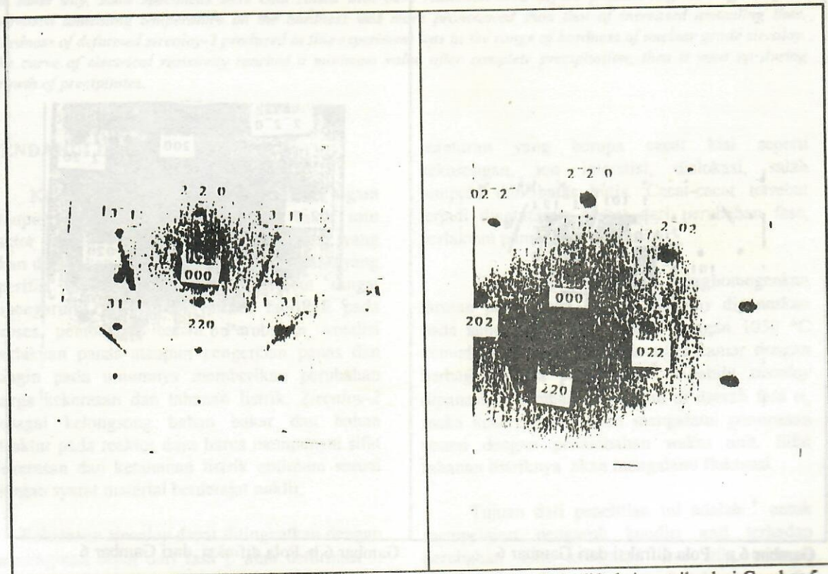
Gambar 5a. Pola difraksi dari Gambar 5
