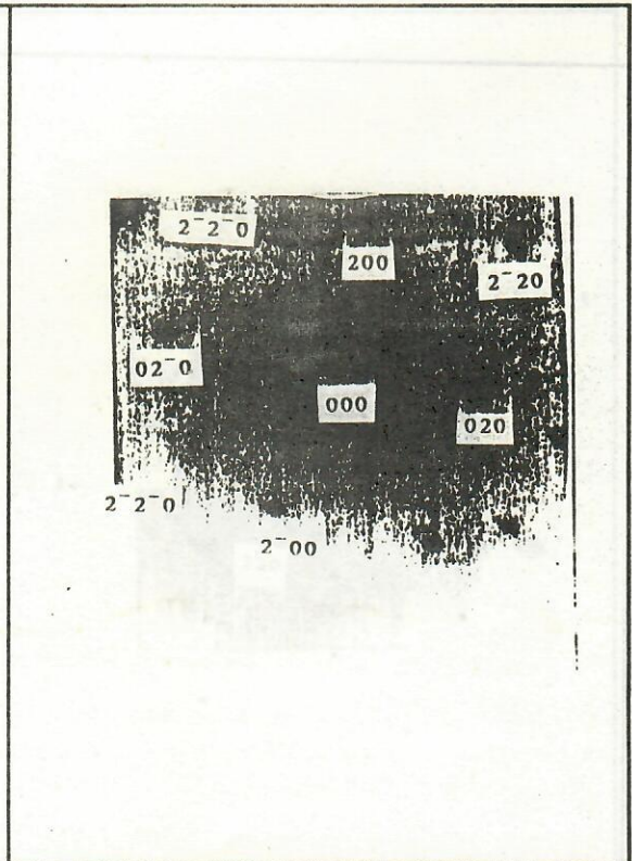
Gambar 6.b. Pola difraksi dari Gambar 6
