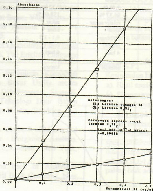
Gambar 3. Kurva kalibrasi analisis silikon dalam U_xSi_2 dengan menggunakan metoda spektrofotometri UV-VIS
