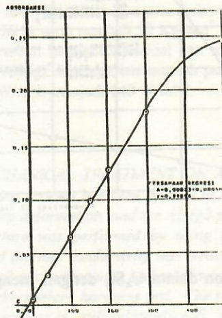
Gambar 1. Kurva absorbansi versus Cadd untuk analisis kadar silikon dalam U_3Si_4 dengan metoda AAFS
