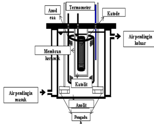
Gambar.1 Bagan sistem elektrokimia pembangkitan oksidator Ag^{+2}
