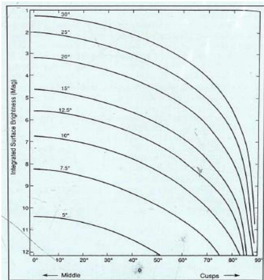
Gambar 3.1. Kurva kuat cahaya sabit bulan. Semakin dekat ke arah matahari (dinyatakan dalam derajat di masing-masing kurva), kuat cahaya semakin redup (angka magnitudonya semakin besar), dan semakin ke arah tanduk sabit (Cusps) juga semakin redup.
