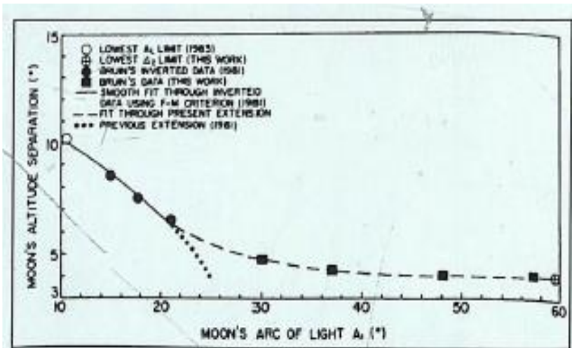
Gambar 3.3. Ilyas (1988) memberikan criteria visibilitas hilal dengan arc of light (beda tinggi bulan-matahari) bergantung pada beda azimuth dengan minimum 4^\circ untuk beda azimuth yang besar dan 10,4^\circ untuk beda azimuth 0^\circ .
