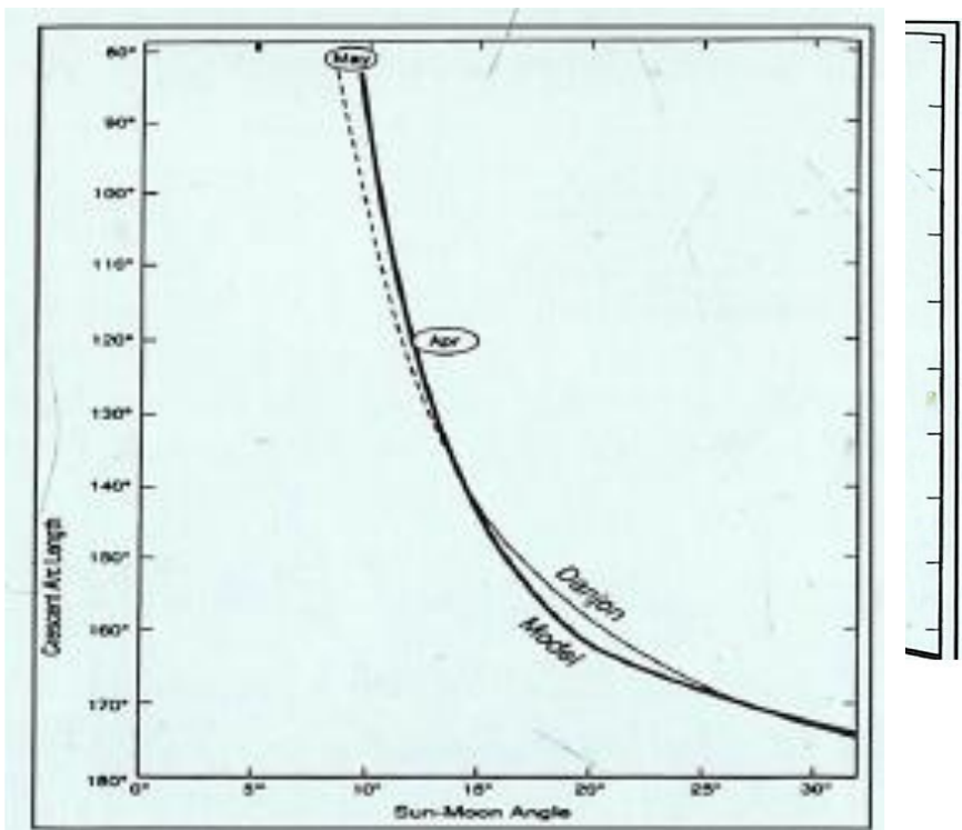
Gambar 3.2. Perbandingan limit Danjon dari hasil ekstrapolasi dengan pengamatan dibandingkan dengan model (Scafer, 1991). Ekstrapolasi jarak sudut bulan-matahari ( Sun-Moon Angle ) pada besar busur hilal ( crescent arc length ) 0^\circ merupakan limit Danjon sekitar 7^\circ .
