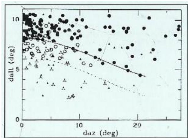
Gambar 3.4. Dari data SAAO, Caldwell dan Laney (2001) memliuat kriteria visibilitas hilal dengan memisahkan pengamatan dengan mata telanjang (bulatan hitam) dan dengan alat bantu optik (bulanan putih). Secara umum, syarat minimal beda tinggi bulan-matahari ( dalt ) > 4^\circ .
